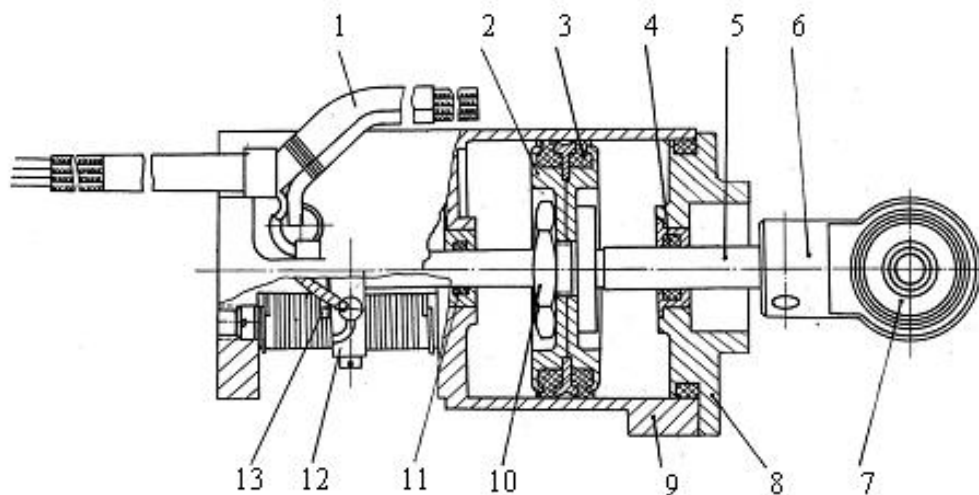
Рис. 40. Рулевая машина: 1 – электрожгут; 2 – диск; 3 – резиновая манжета; 4,11 – уплотнительные кольца; 5 – шток; 6 – серьга; 7 – подшипник; 8 – крышка; 9 – корпус; 10 – гайка; 12 – потенциометр обратной связи; 13 – контактная пластина; 14 – движок потенциометра
