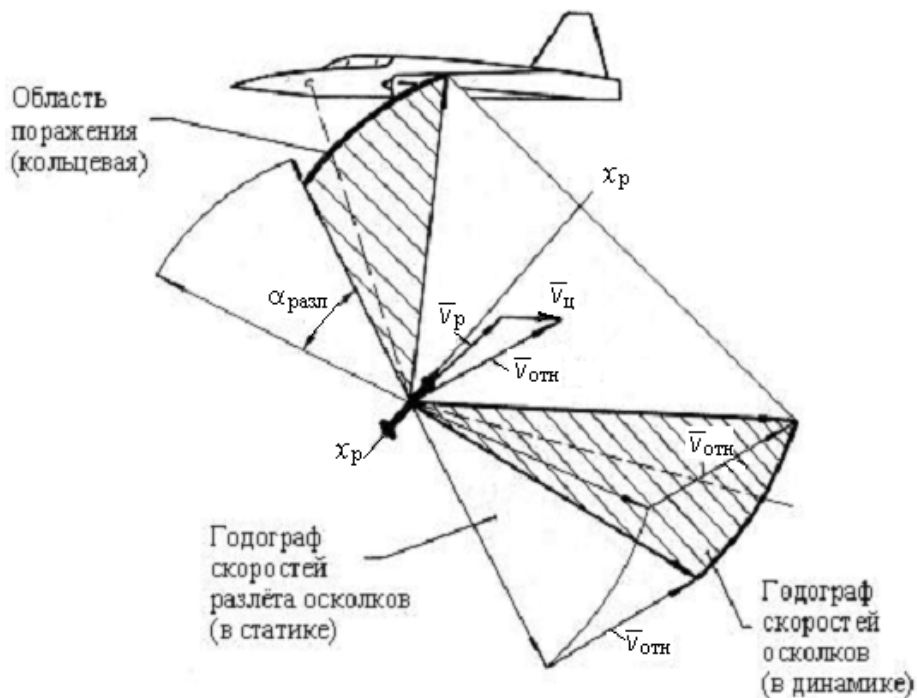
Рис. 33. Кинематическая схема накрытия цели областью поражения БЧ: - - - - линия срабатывания радиовзрывателя; x_p – продольная ось ракеты; \alpha_{\text{разл}} – угол разлета осколков; \bar{V}_p, \bar{V}_ц, \bar{V}_{\text{отн}} – скорость ракеты, цели и относительная скорость
