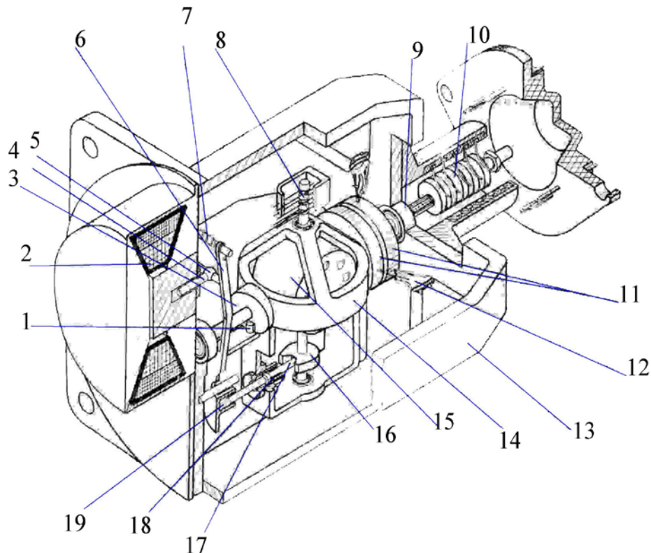
Рис. 26. Конструкция свободного гироскопа: 1 – ролик; 2 – катушка электромагнита; 3 – кулачок; 4 – подвижный якорь; 5 – серьга; 6 – рычаг; 7 – пружина; 8 – коллекторное кольцо на оси внутренней рамки; 9 – подшипник; 10 – коллекторное кольцо на оси внешней рамки; 11 – потенциометр; 12 – контактная щетка; 13 – корпус; 14 – внешняя рамка; 15 – внутренняя рамка; 16 – профилирующий кулачок на оси внутренней рамки; 17 – толкатель; 18 – пружина; 19 – ловитель
